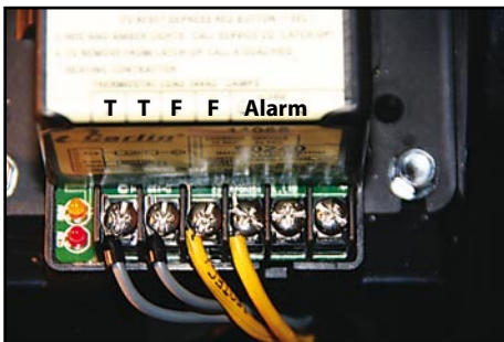
Контролер горелки
